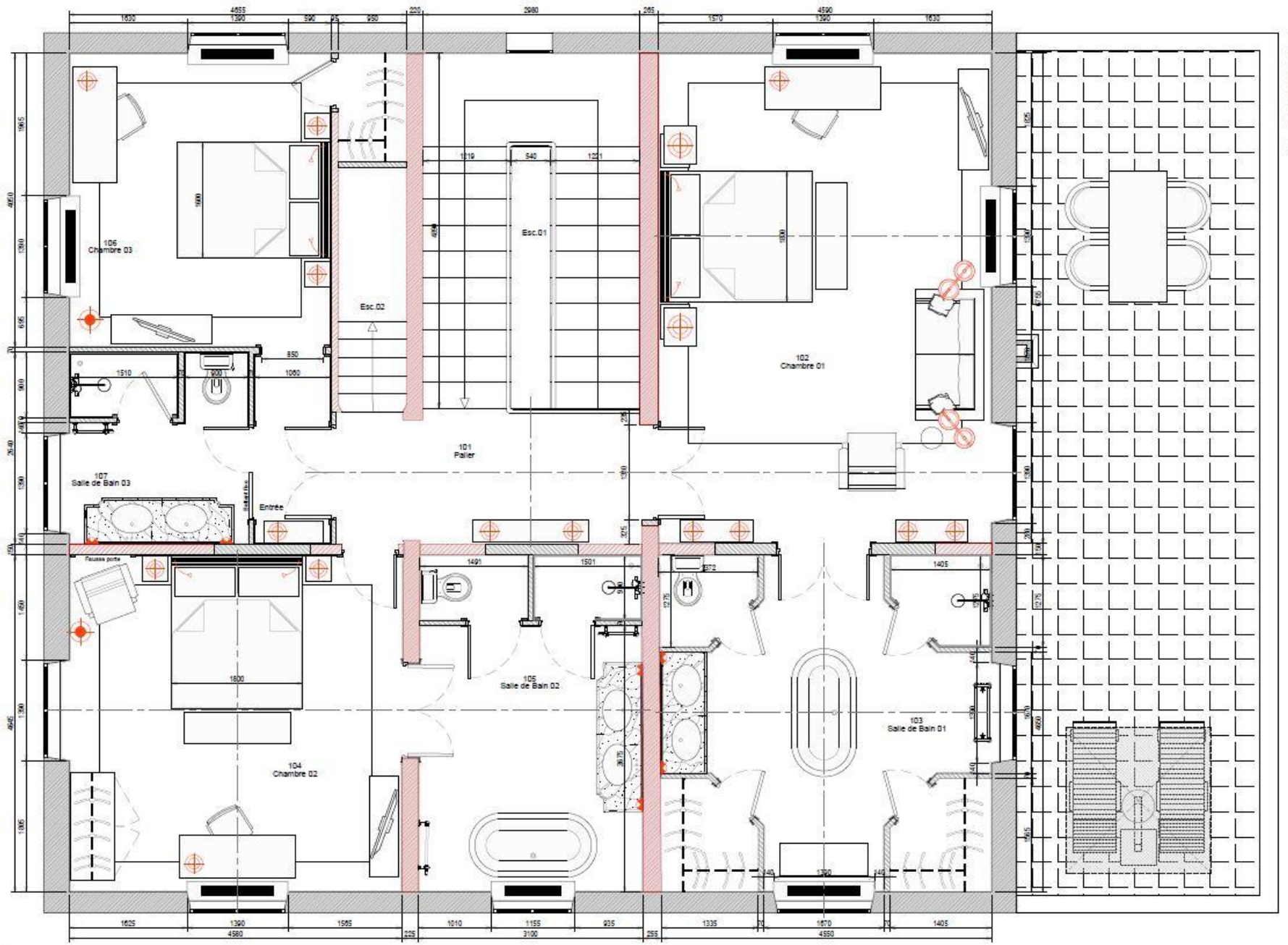
CASA PRINCIPAL, PLANTA PRIMERA
