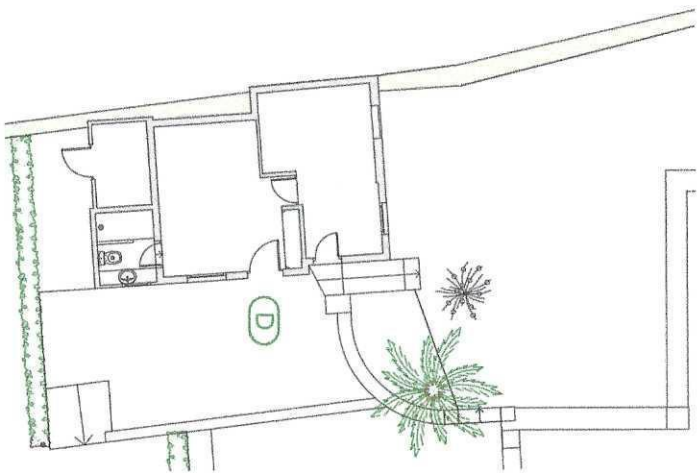
PLANTA DEFINITIVA EDIFICIO D
