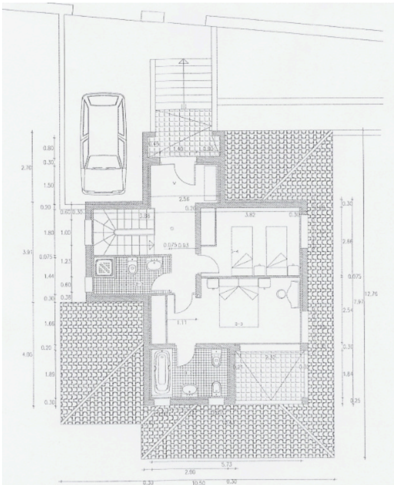
PLANTA PISO
