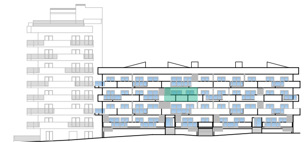
Alçado Sul
